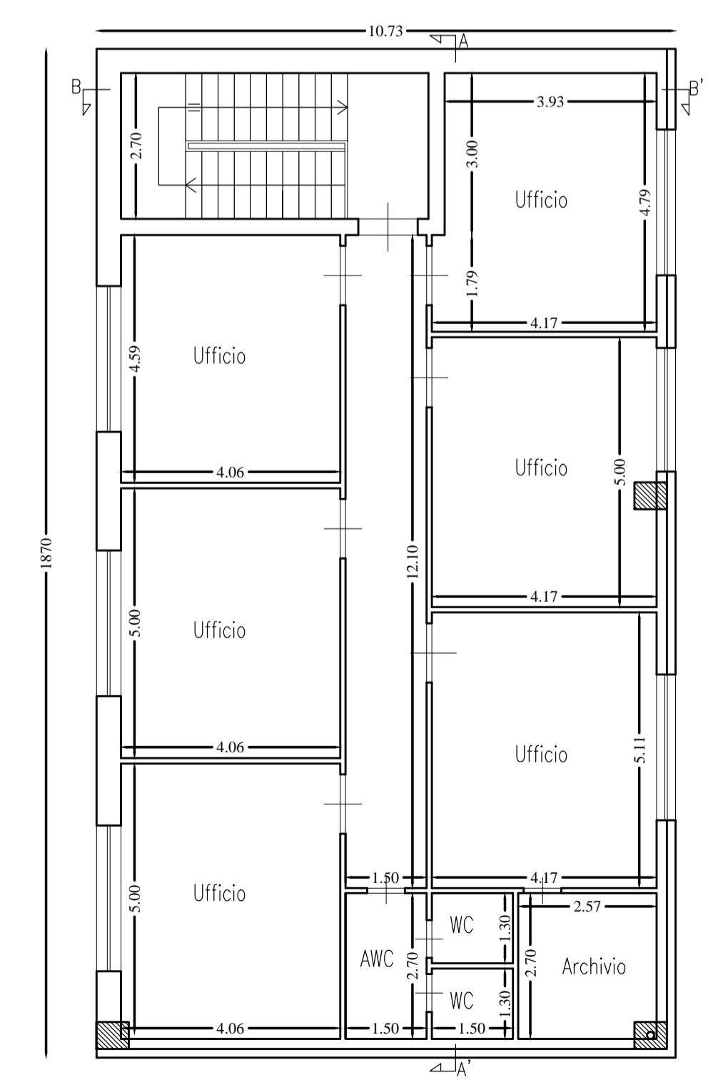
PIANTA PRIMO PIANO - SCALA 1:100
