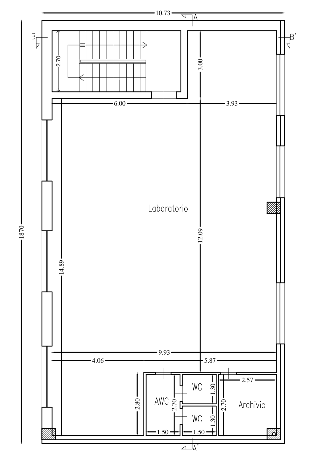
PIANTA SECONDO PIANO - SCALA 1:100
