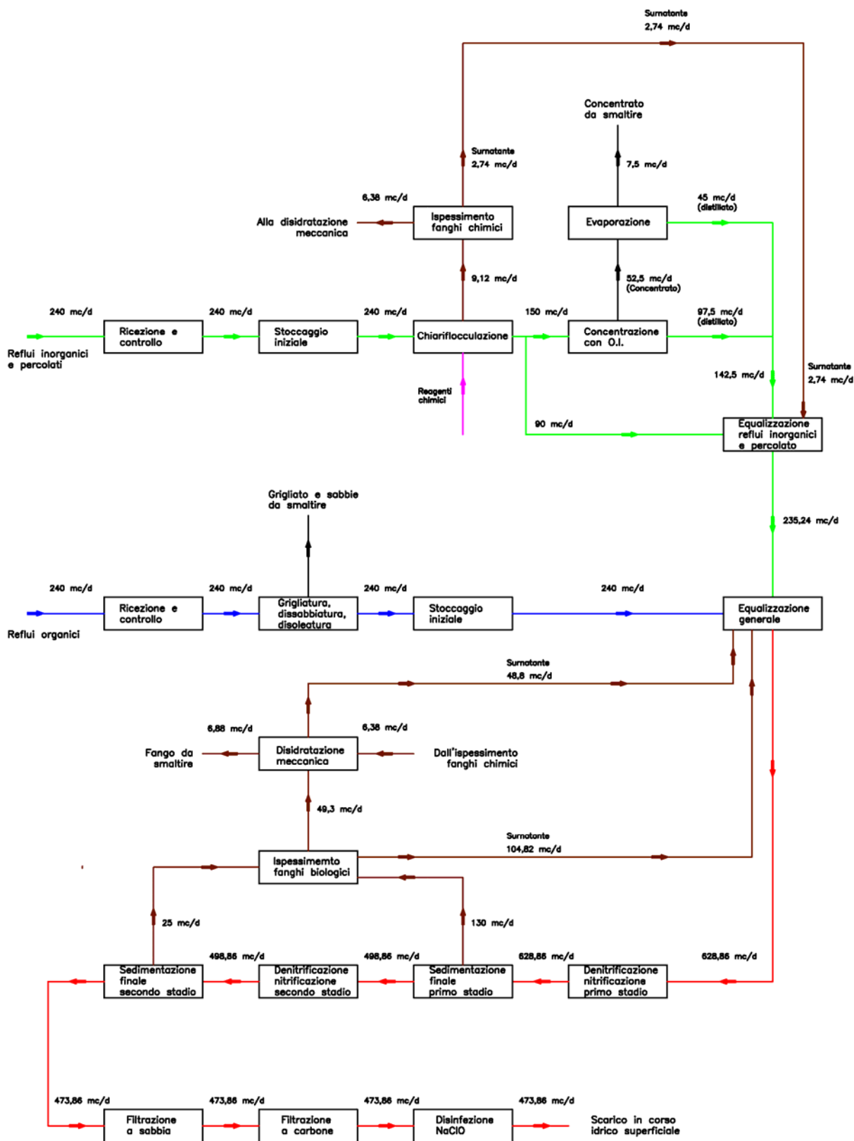
Figura 3.1. Schema a Blocchi di funzionamento dell'impianto
